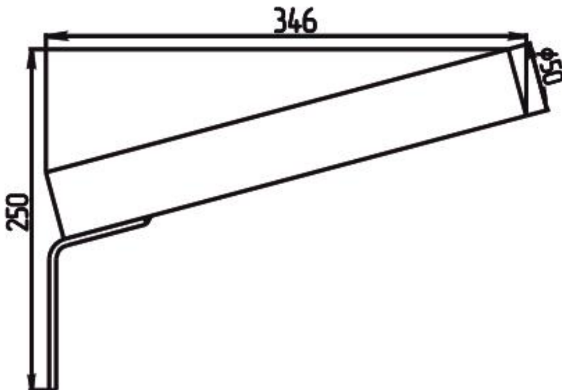
Рисунок 1 - Внешний вид и габаритные, присоединительные размеры кронштейна КР-2М
