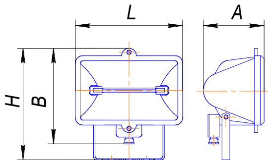
Рис. 1. Общий вид прожектора ИО 04-150/200/300/500-01.
