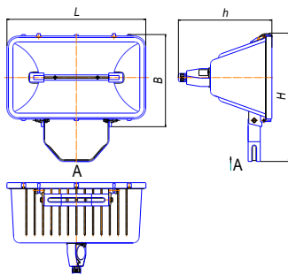
Рис.1 Общий вид прожектора ИО 01-2000-07
