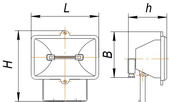
Рис. 1. Общий вид прожектора ИО 02-500-001.
